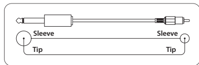
Рис. 5.1: Разводка Mono-кабеля
