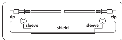
Рис. 5.1: Разводка Cinch-кабеля
